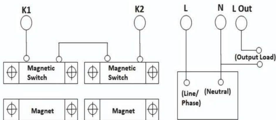
1L-AC101SD-DOUBLE DOOR CONNECTION DIG.
